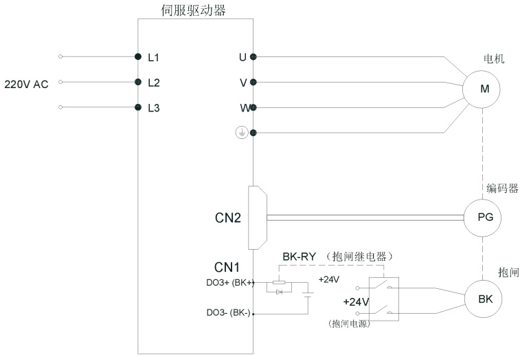
图 6-3 抱闸配线图
