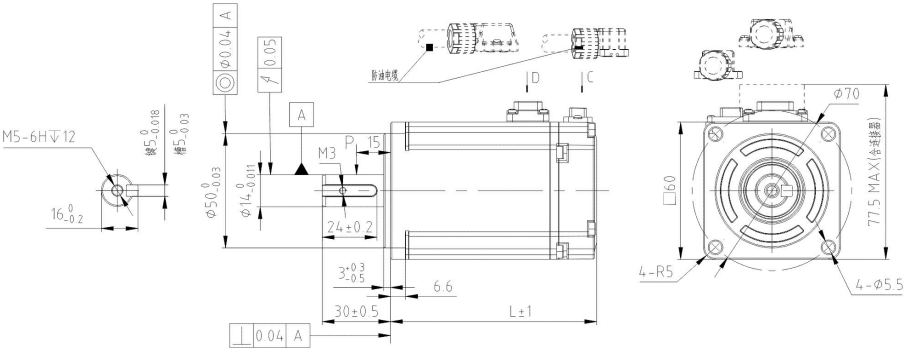
图 2-10 60 框号中惯量伺服电机（ST4-L 系列）外形尺寸图
