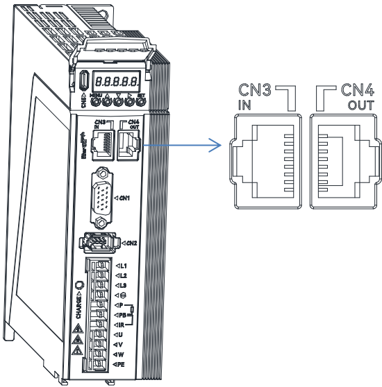
图 4-12 通讯接口连接图
