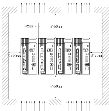
紧凑安装
