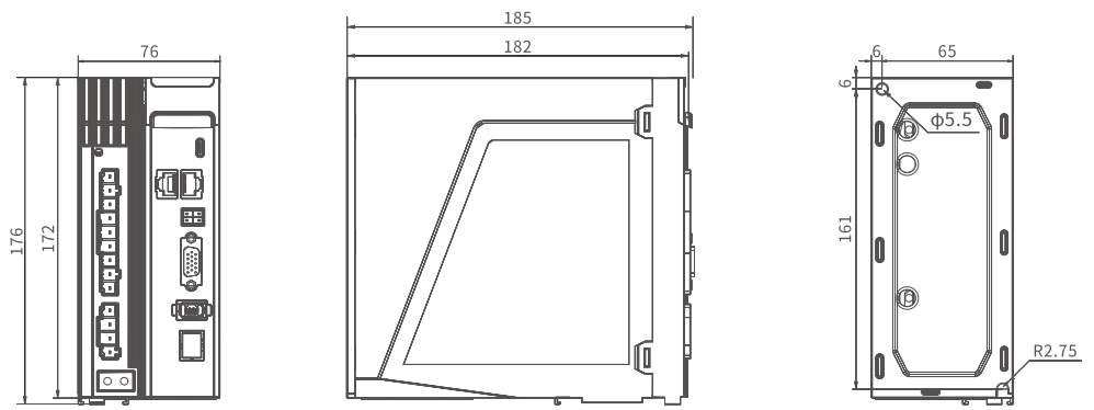
图 2-3 SIZE D 伺服驱动器外形尺寸图
