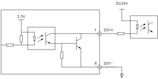
图 4-10 DO 端子漏型 (NPN) 输出接线方式
