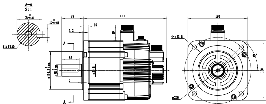
图 2-13 180 框号中惯量伺服电机（W 系列）外形尺寸图
