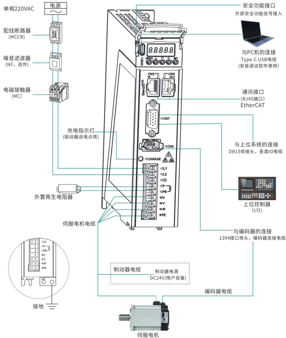
图 3-4 SIZE A 单相 220V 伺服系统配线图
