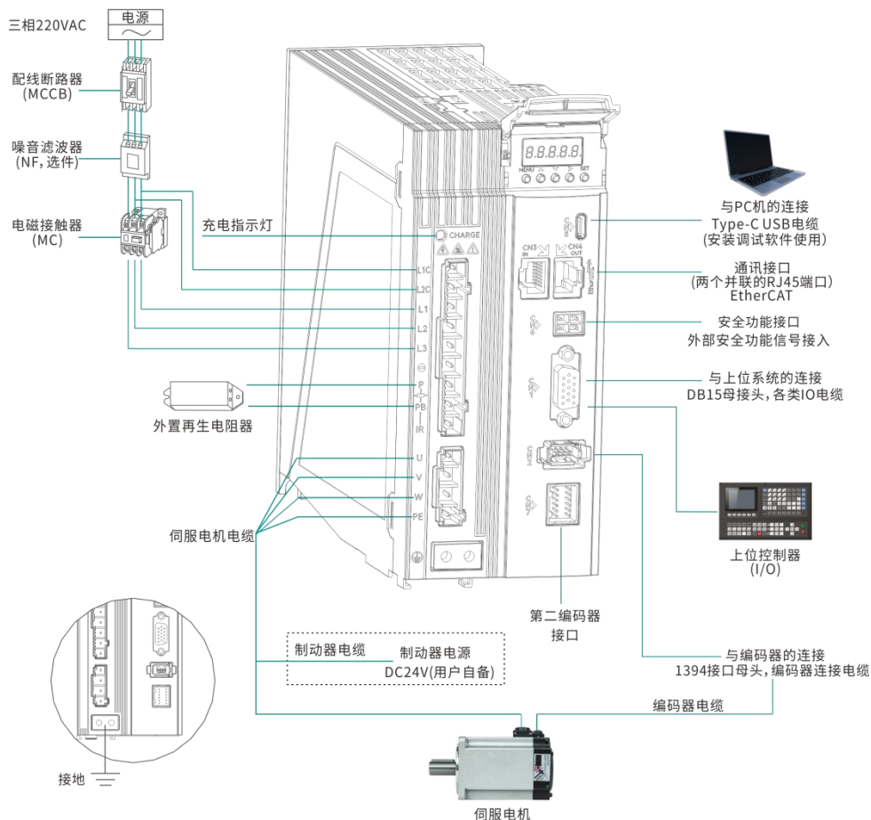
图 3-6 SIZE D 三相 220V 伺服系统配线图
