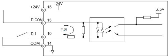
图 4-3 DI 端子干接点连接方式（使用伺服驱动器内部 24V 电源）
