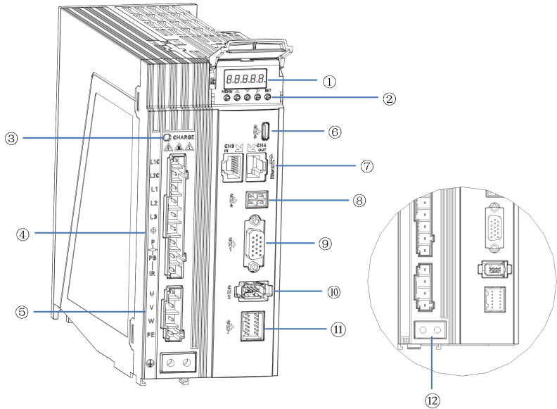
图 1-7 M5-N 伺服驱动器各部分示意图 (M5-NS012A、M5-NS016A、M5-NT3R5A、M5-NT5R4A、M5-NT8R4A、M5-NT012A)
