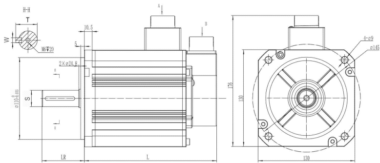
图 2-12 130 框号中惯量伺服电机（W 系列）外形尺寸图
