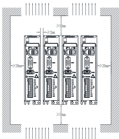
紧凑安装
