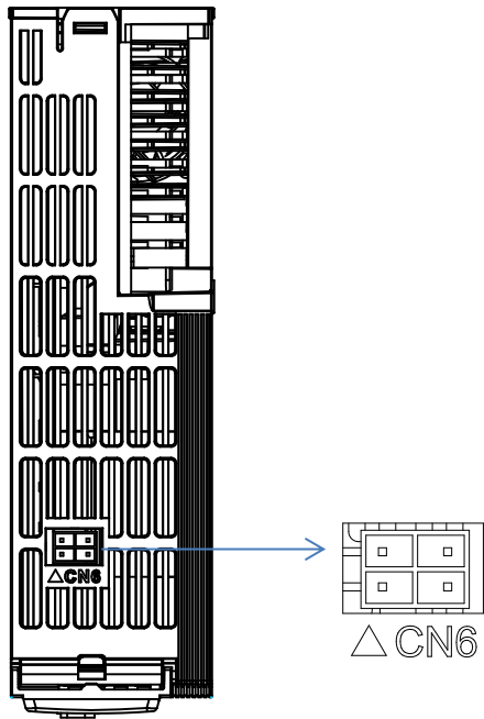
图 4-13 STO 端子接线图
