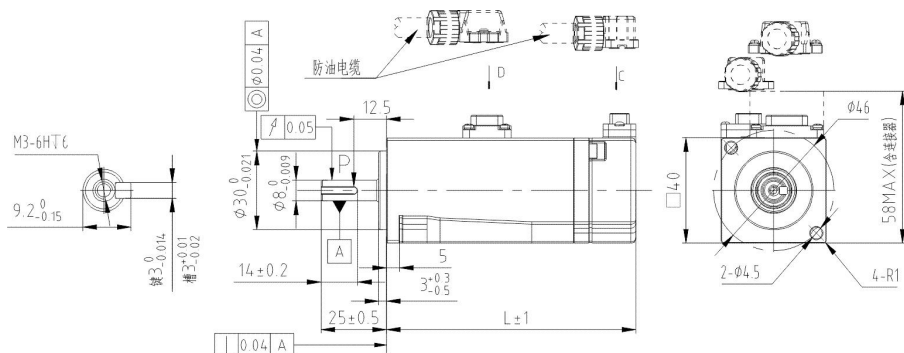
图 2-7 40 框号中惯量伺服电机（ST1-L 系列）外形尺寸图
