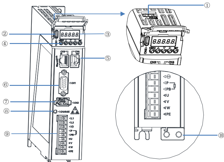
图 1-5 M5-N 伺服驱动器各部分示意图（M5-NS1R6A、M5-NS2R8A）
