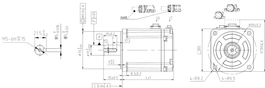
图 2-11 80 框中惯量伺服电机（ST4-L 系列）外形尺寸图
