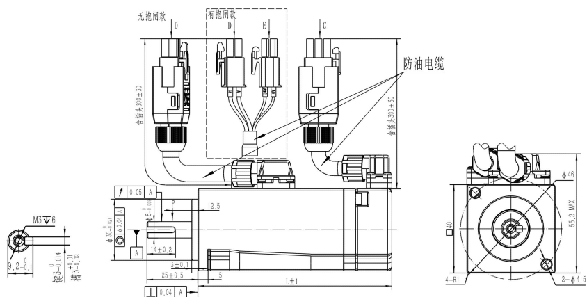
图 2-4 40 框号中惯量伺服电机 (L 系列) 外形尺寸图
