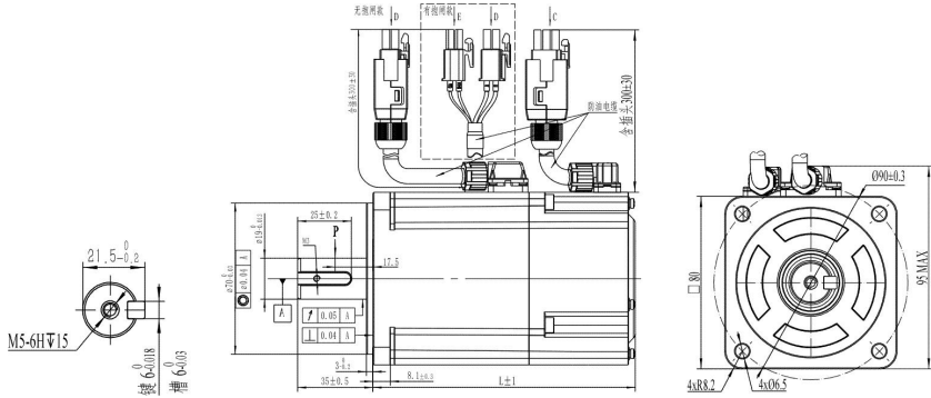
图 2-6 80 框号中惯量伺服电机（L 系列）外形尺寸图
