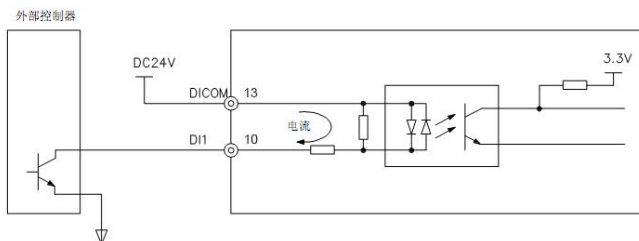
图 4-6 DI 端子 NPN 连接方式 (使用外部电源)
