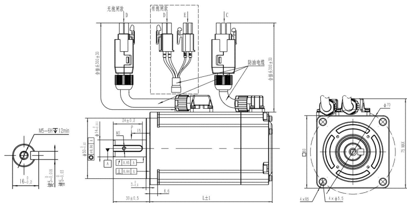
图 2-5 60 框号中惯量伺服电机 (L 系列) 外形尺寸图
