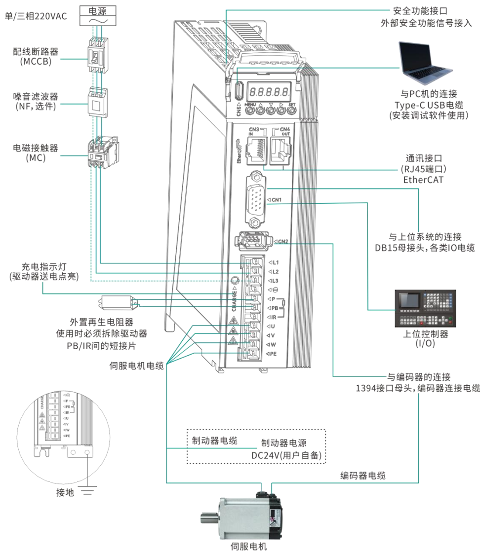
图 3-5 SIZE B 单/三相 220V 伺服系统配线图
