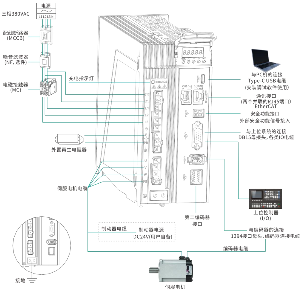
图 3-7 SIZE D 三相 380V 伺服系统配线图
