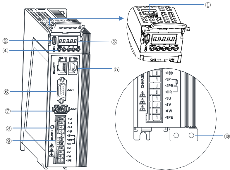
图 1-6 M5-N 伺服驱动器各部分示意图（M5-NS5R5A、M5-NS7R6A）
